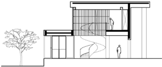
大堂立面图
